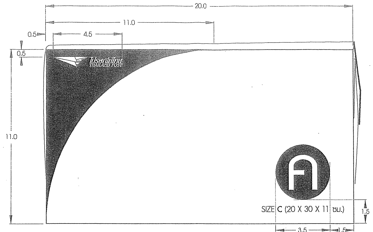
รูปด้านข้าง (ซ้าย) มาตราส่วน 1:1.25
