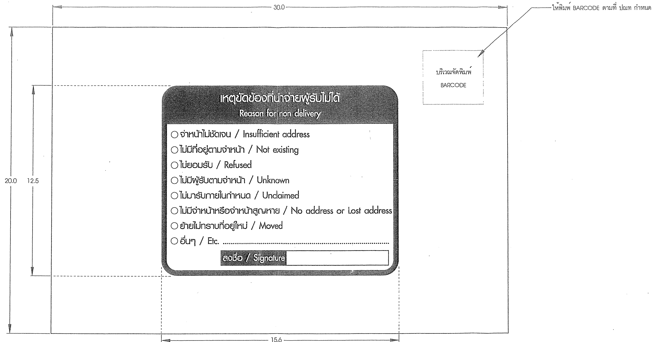
รูปด้านล่าง (กันล่อง) มาตราส่วน 1:1.25
