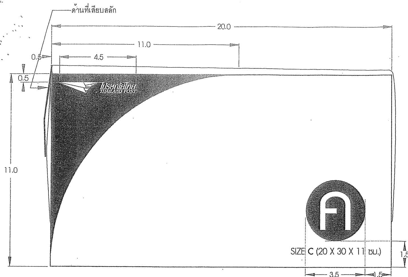
รูปด้านข้าง (ขวา) มาตราส่วน 1:1.25
