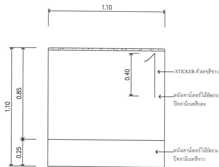
รูปด้าน 1 มาตราส่วน 1:20
