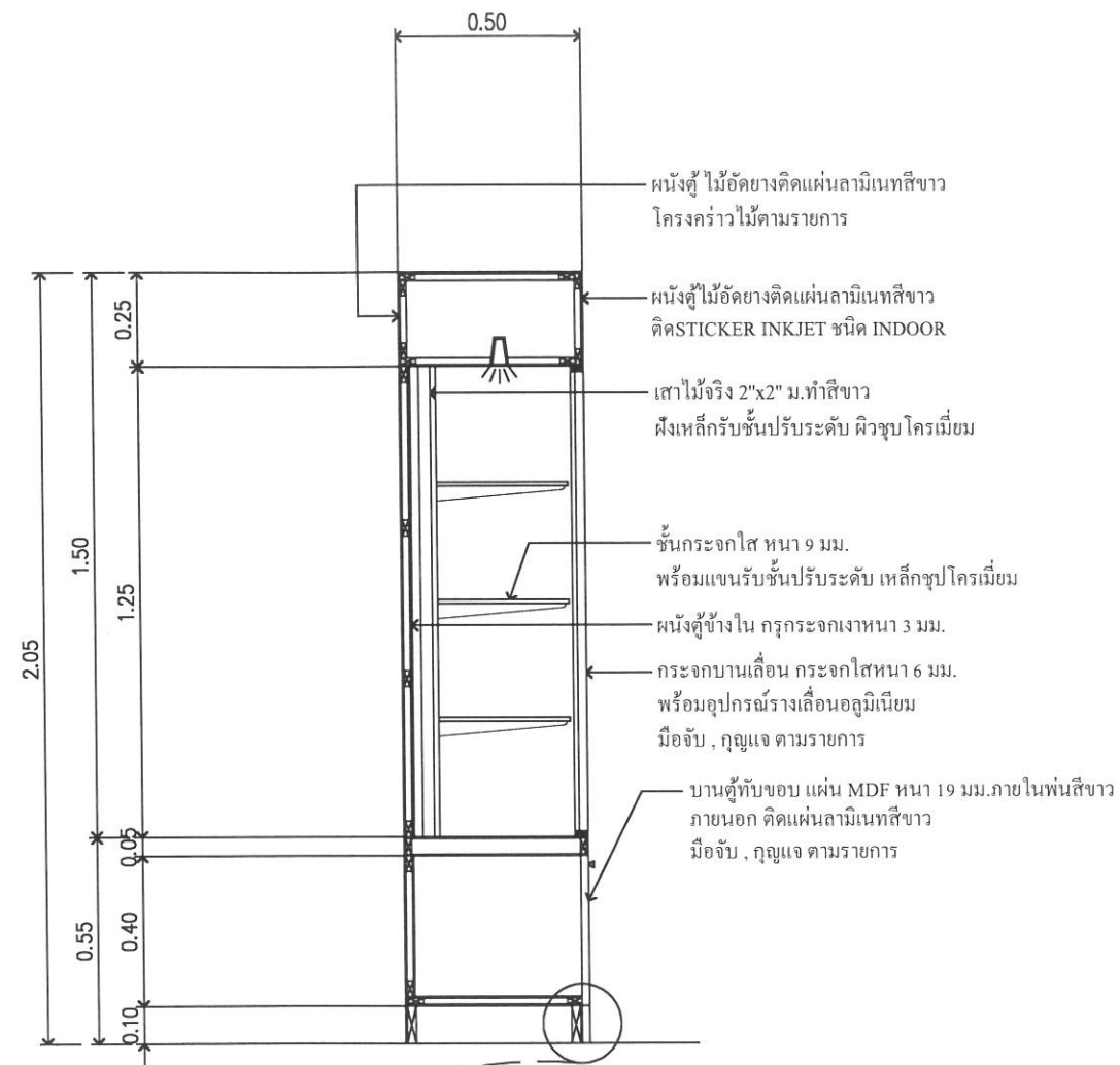
ขอบล่าง ไม้สัก 1"x4" ติดแผ่นลามิเนทสีเทา
