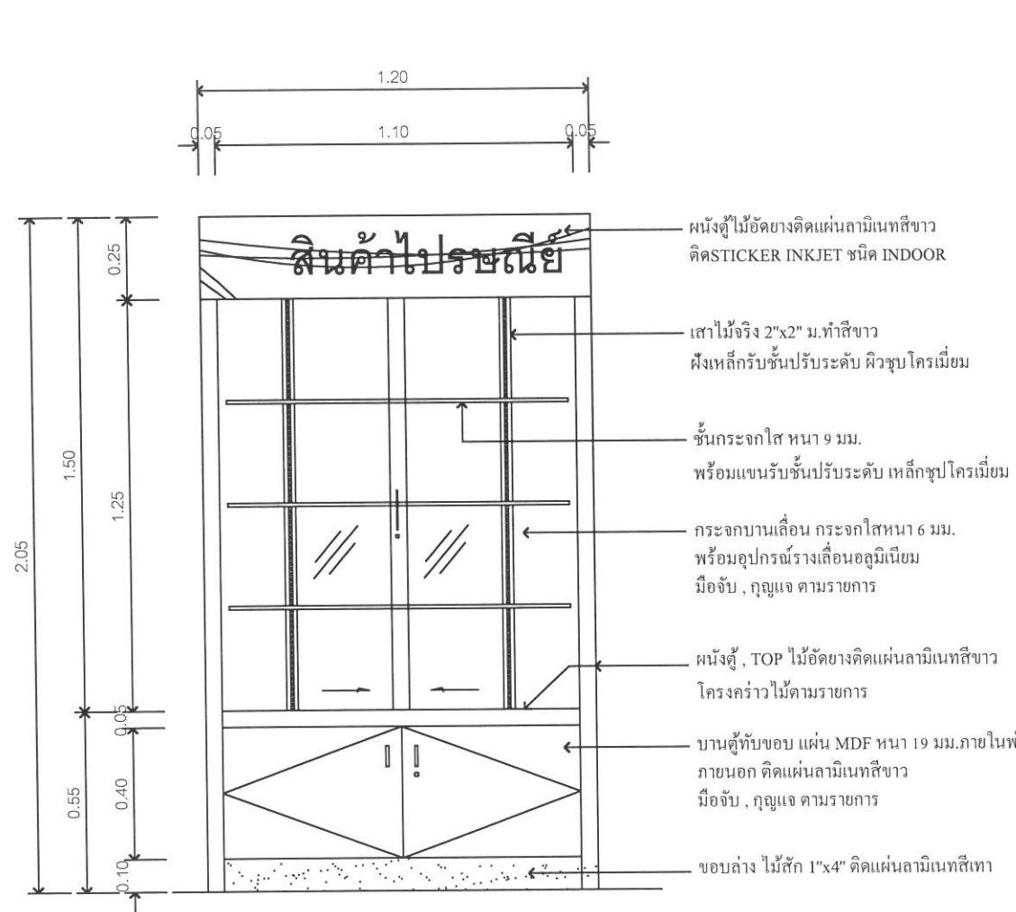
รูปด้าน 1 มาตราส่วน 1:20
