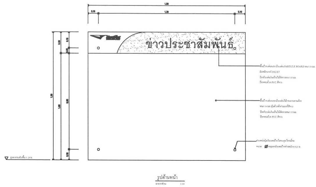
B4 แบบขยายป้ายประชาสัมพันธ์
