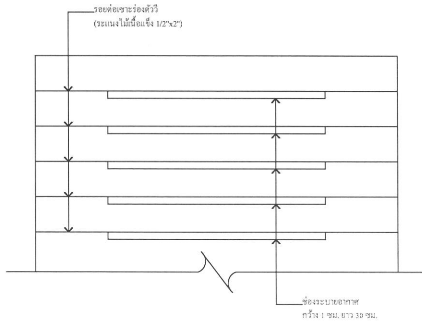
ขยายช่องระบายอากาศ มาตราส่วน 1:5
