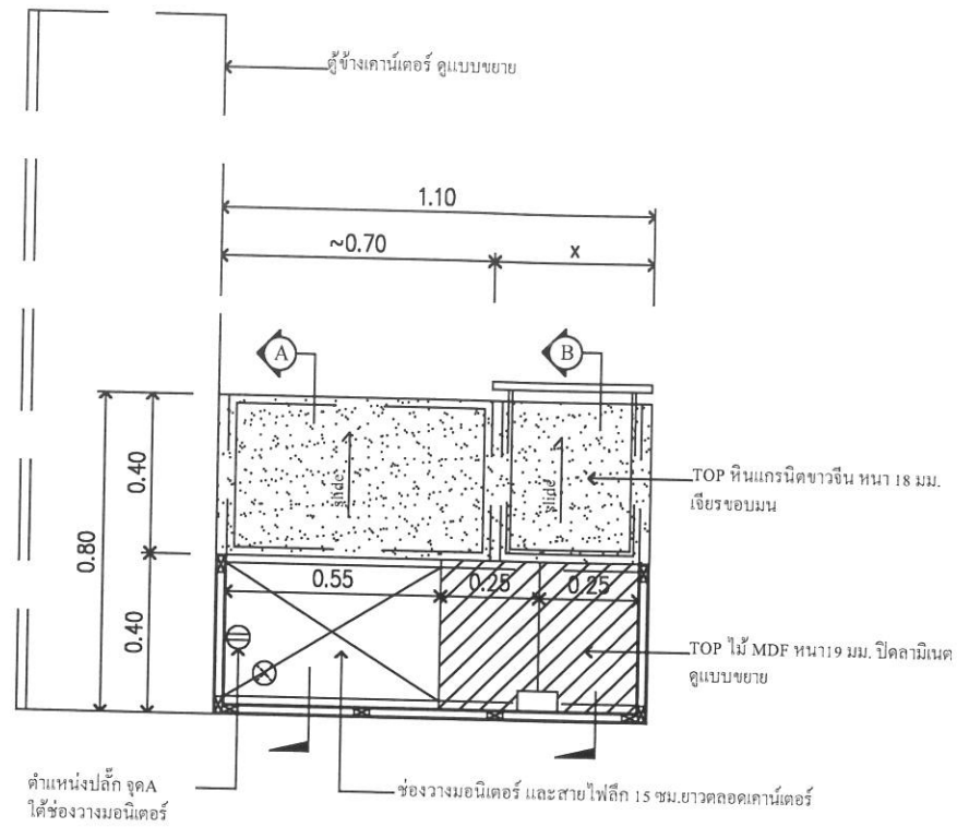
แปลนเคาน์เตอร์บริการ CA POS (ส่วนล่าง) มาตราส่วน 1:20
