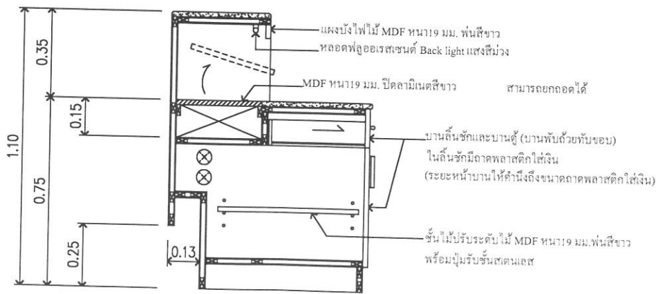
รูปตัด B มาตราส่วน 1:20
