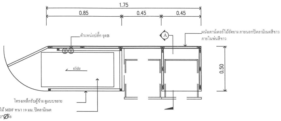
แปลนตู้ข้างเคาน์เตอร์บริการ CA POS (ส่วนล่าง) มาตราส่วน 1:20
