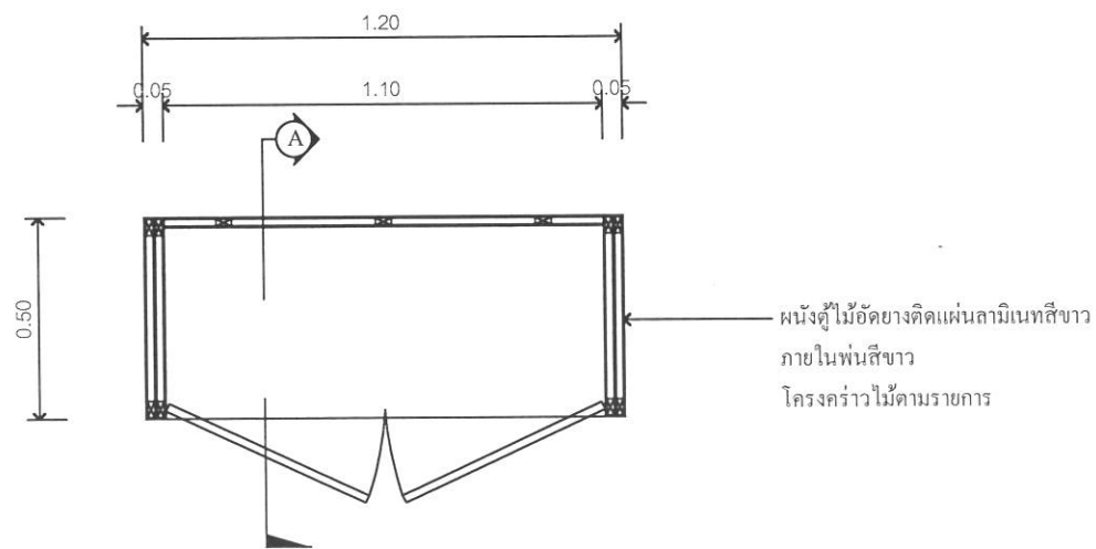
แปลนตู้โชว์สินค้าไปรษณีย์ (ส่วนล่าง)
