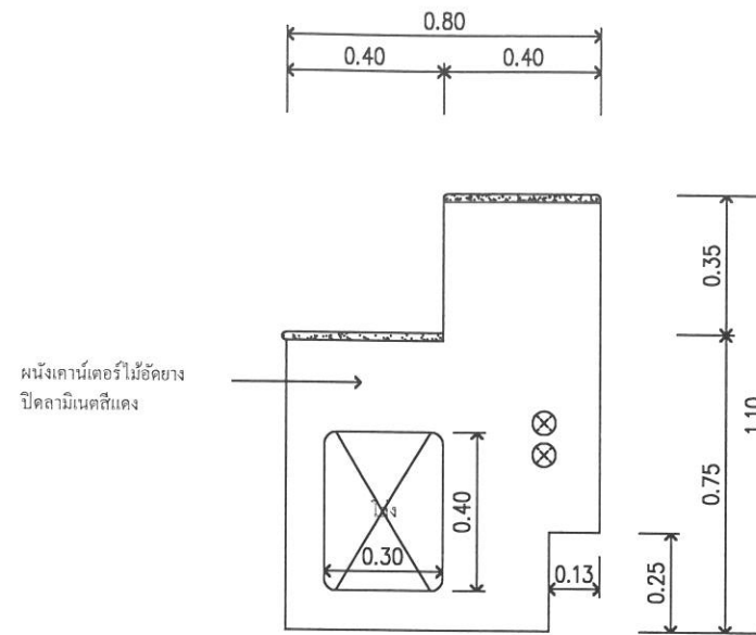
รูปด้าน 2 มาตราส่วน 1:20
