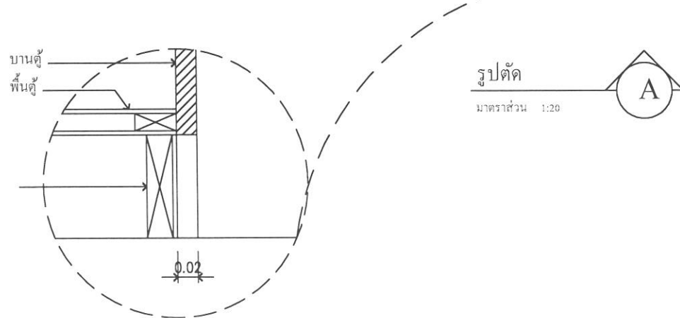
ขอบล่าง ไม้สัก 1"x4" ติดแผ่นลามิเนทสีเทา
