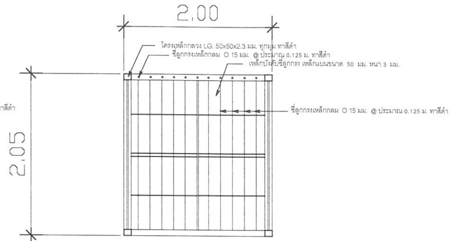
แบบ F-4 Not to Scale
