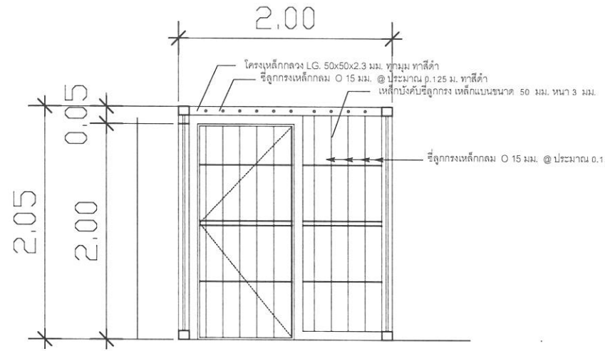
รูปด้านหน้า Not to Scale
