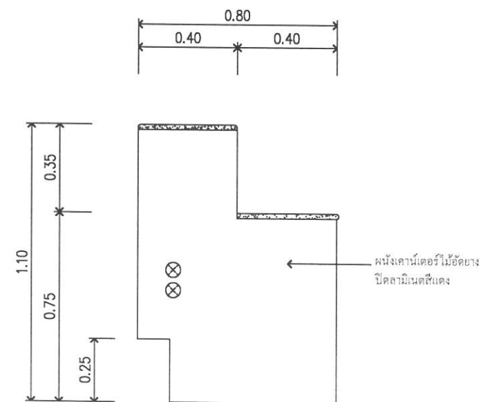
รูปด้าน 4 มาตราส่วน 1:20
