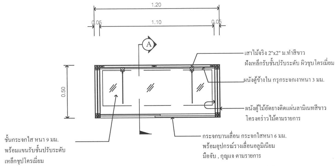
แปลนตู้โชว์สินค้าไปรษณีย์
