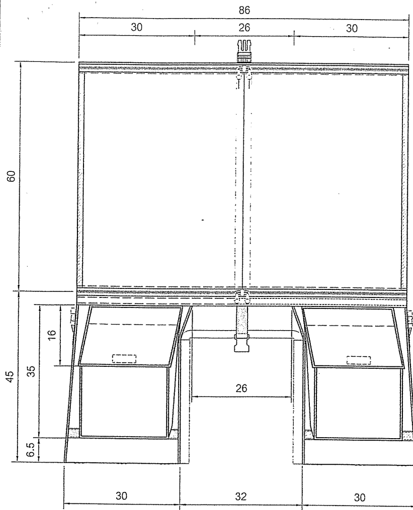
รูปด้านหน้า มาตราส่วน 1 : 10
