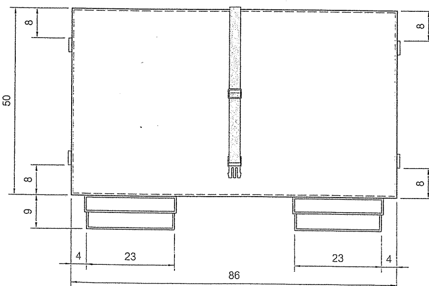
รูปด้านบน มาตราส่วน 1 : 10
