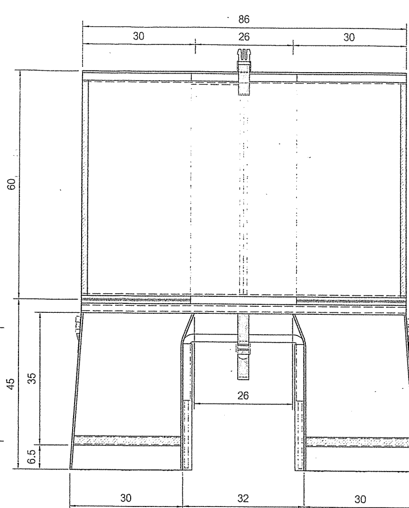
รูปด้านหลัง มาตราส่วน 1 : 10
