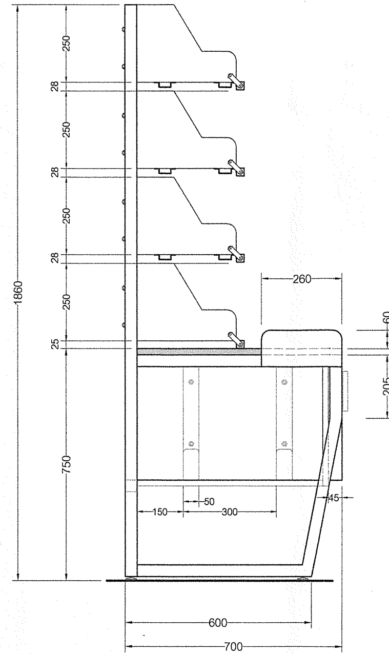
รูปด้านข้างขวา มาตราส่วน 1 : 12.5
