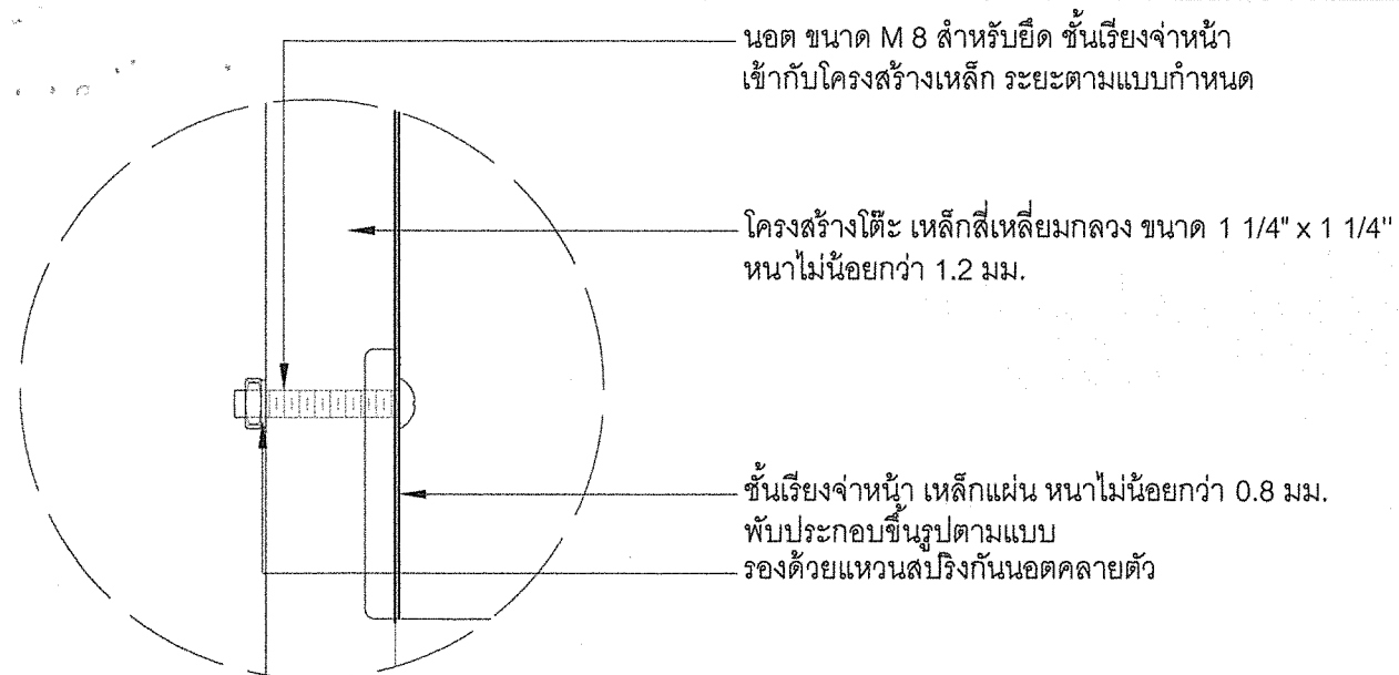
รูปขยาย ①
