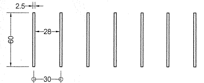
รูปขยาย ④ มาตราส่วน 1 : 2.5
