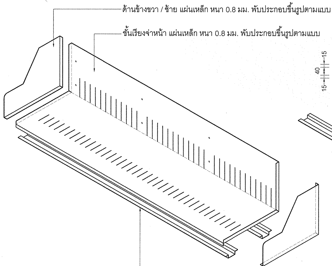
ภาพคลี่แผ่นขึ้นเรียงจำหน่าย มาตราส่วน 1 : 10
