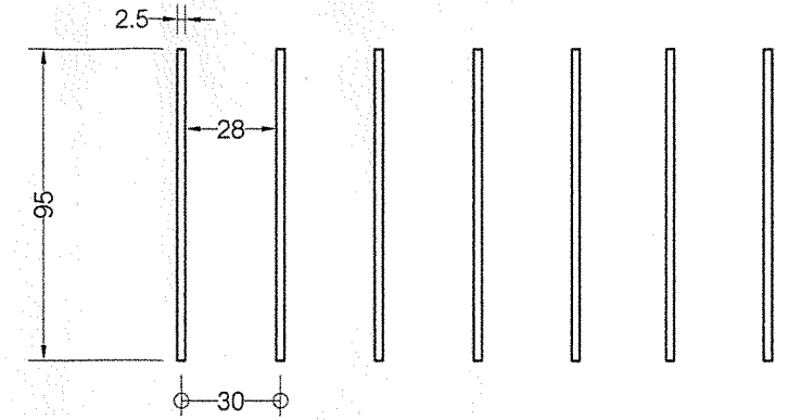
รูปขยาย ③ มาตราส่วน 1 : 2.5
