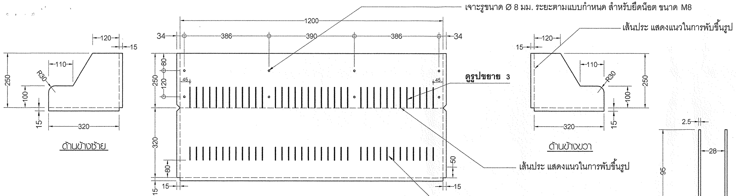
ภาพคลี่แผ่นขึ้นเรียงจำหน่าย มาตราส่วน 1 : 10
