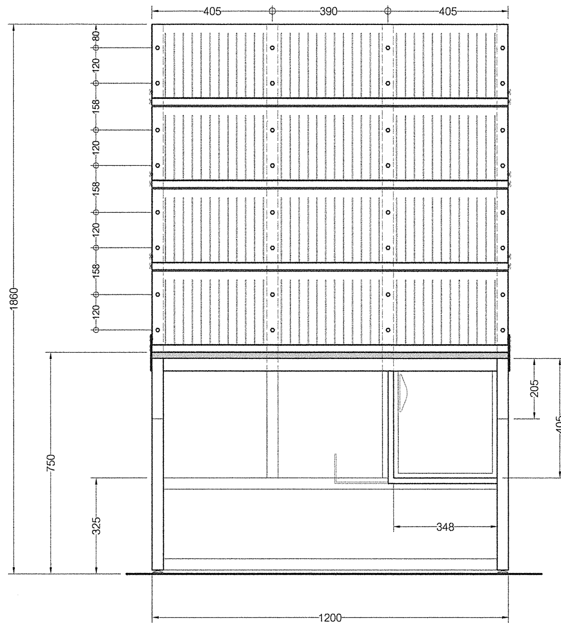
รูปด้านหน้า มาตราส่วน 1 : 12.5
