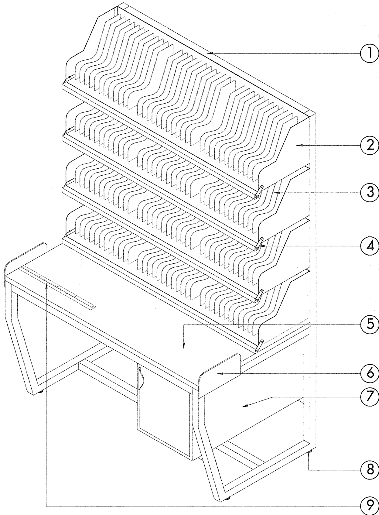
ทัศนียภาพ มาตราส่วน 1:12.5
