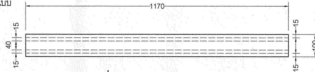
ภาพคลี่คานเสริมความแข็งแรง มาตราส่วน 1 : 10
