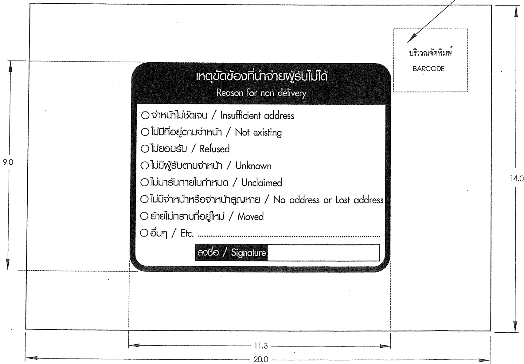
รูปด้านล่าง (ก้นกล่อง) มาตราส่วน 1:1
