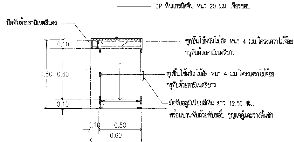
แบบรูปตัด A-A
