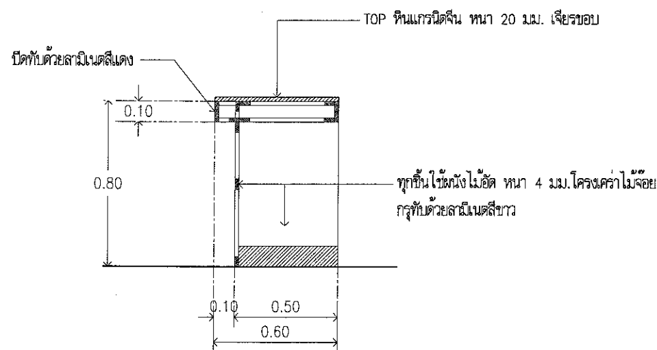
แบบรูปตัด B-B
