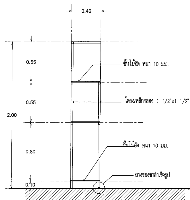
แบบรูปด้าน A ชั้นวางของ
