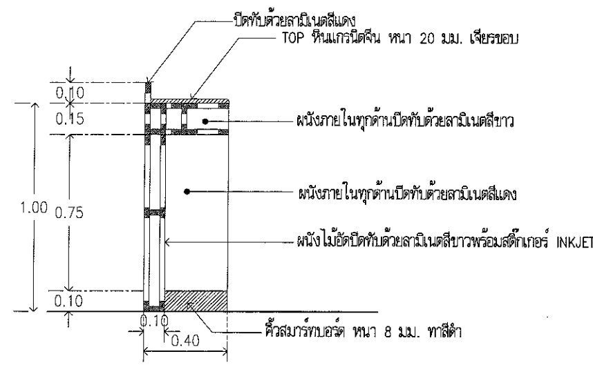
รูปตัด B-B
