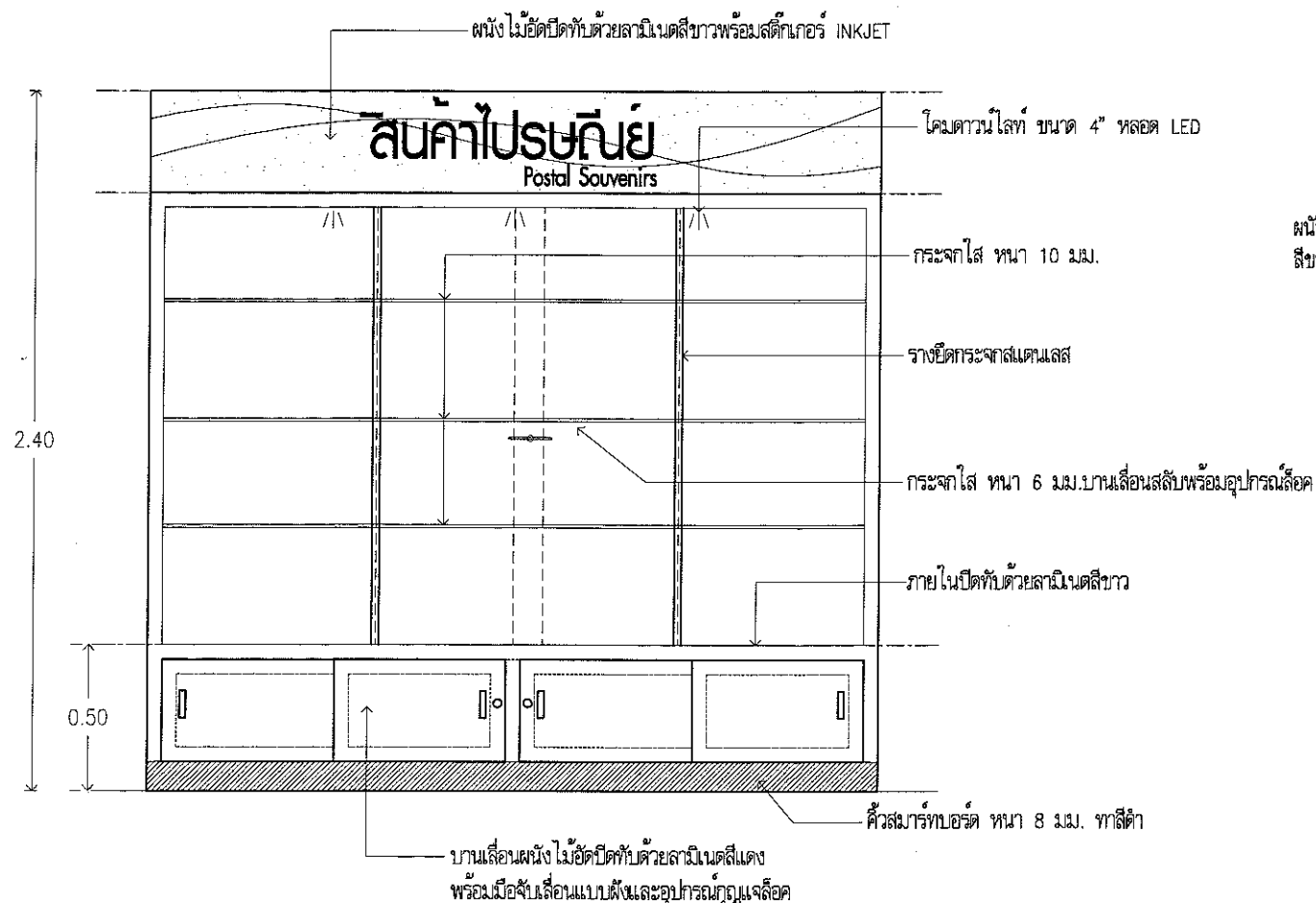
รูปด้านหน้า
