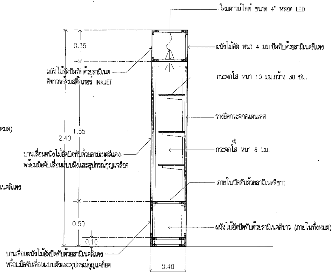
รูปตัด A-A
