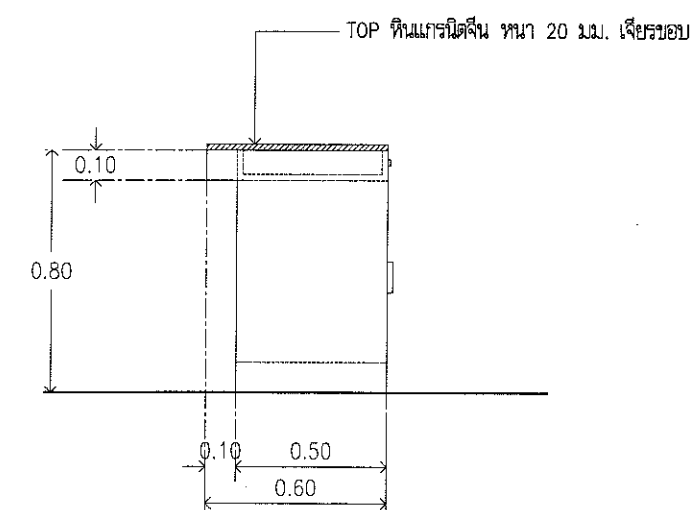
แบบขยายเคาน์เตอร์ภายในกล่องของ/ตู้ห่อ F2
