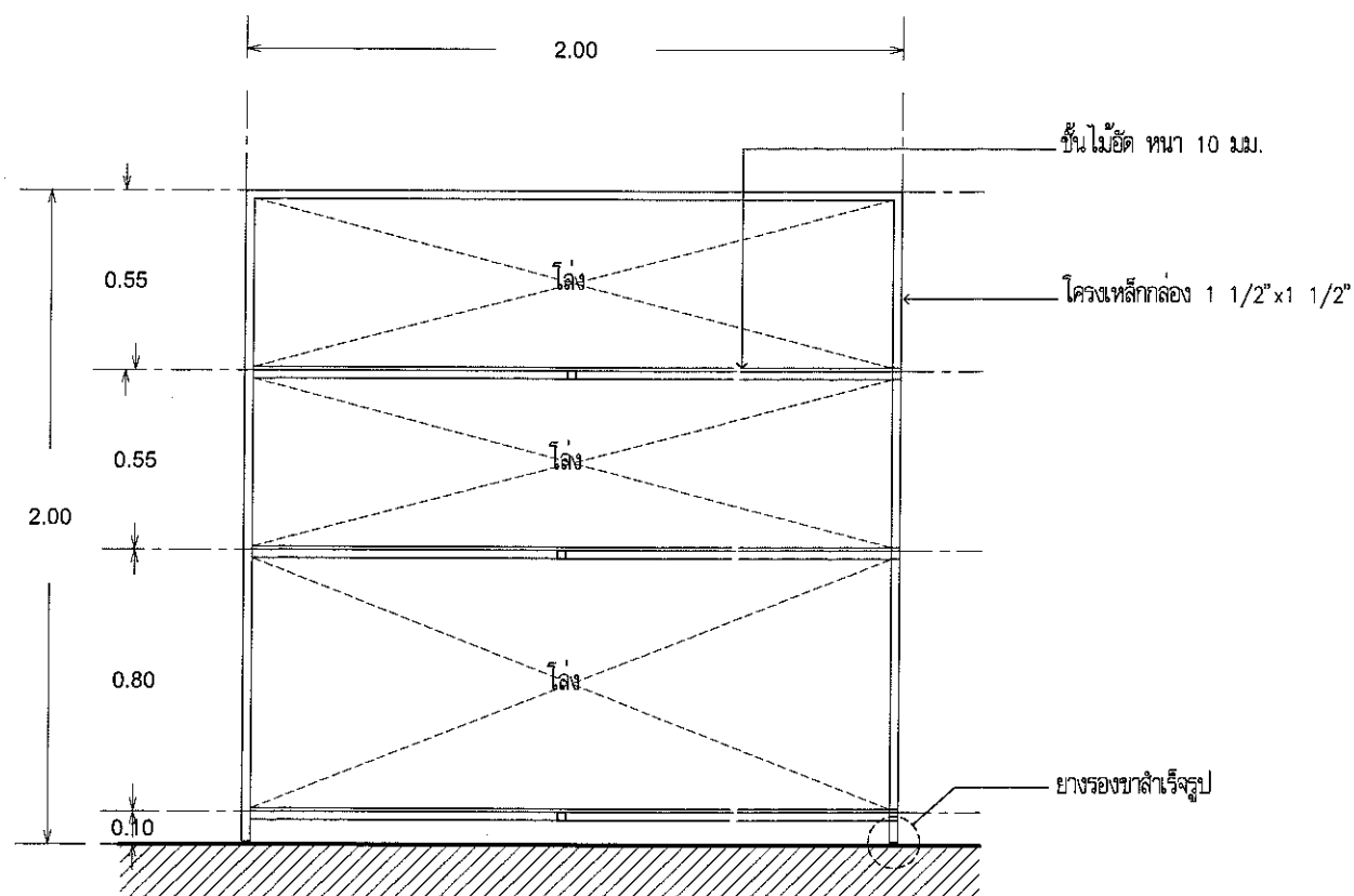
แบบรูปด้าน A ชั้นวางของ
