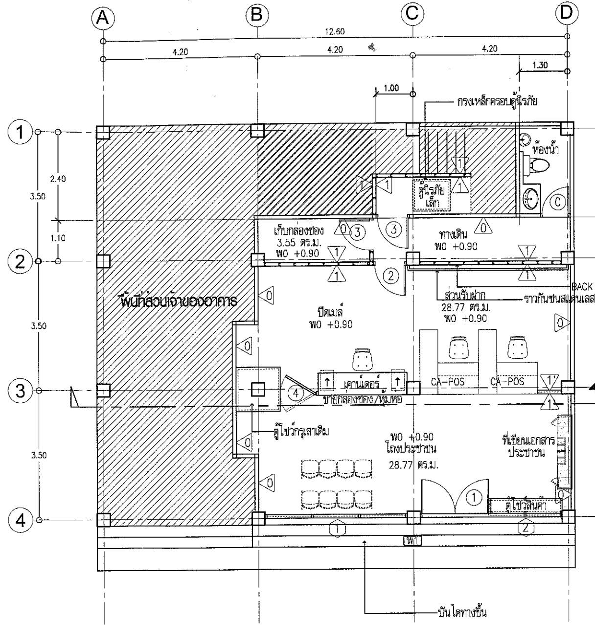
แปลนพื้นที่ (ปรับปรุง) มาตราส่วน 1:100
