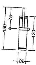
รูปด้านหน้า DOLLY 1:3
